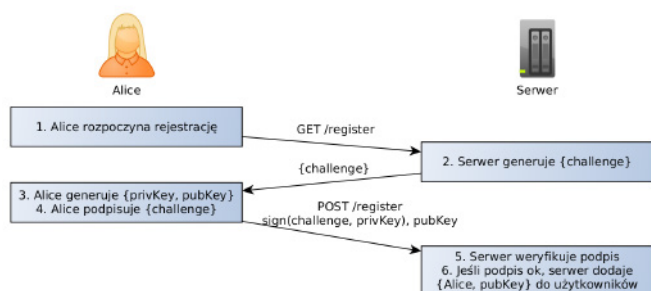
Rysunek 1. Komunikacja klient-serwer podczas przeprowadzania procedury rejestracji
